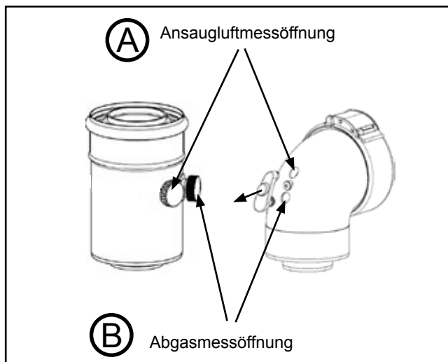
Bild: Messung Ansaugluft und Abgasparameter für Abgassystem 60/100 für optionale Geräteausführung
