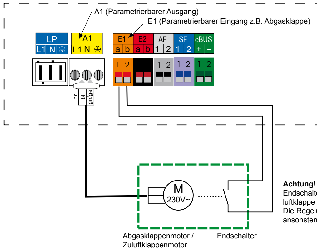
Elektroanschluss HCM-2
