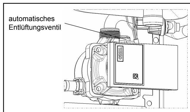
Bild: Automatisches Entlüftungsventil an der Heizkreispumpe
