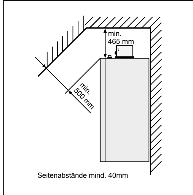
Bild: Mindestabstände
