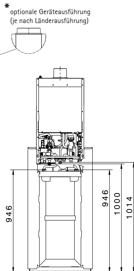
Rückansicht CGS-2R
