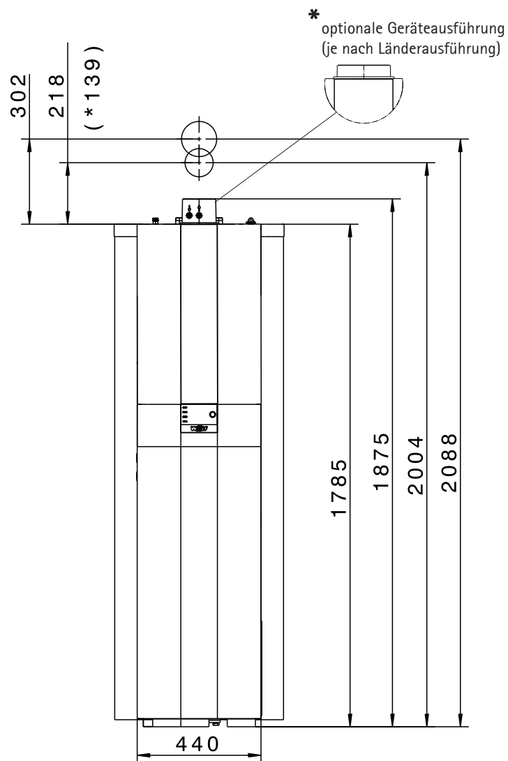
Vorderansicht CSZ-2R
