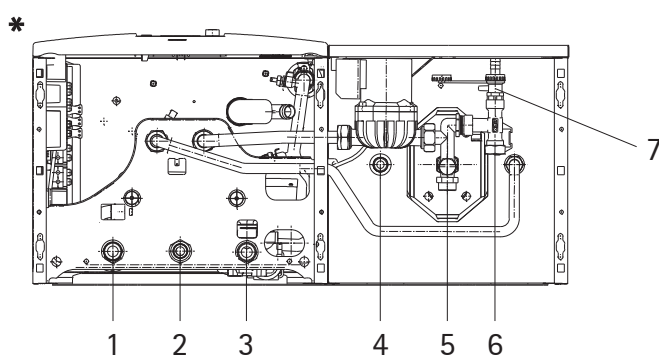
Unteransicht CGW-2
